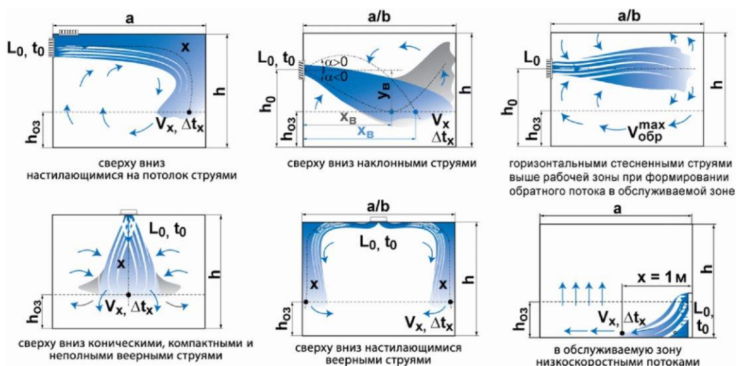
Рисунок Ж.1 - Основные схемы подачи приточного воздуха
